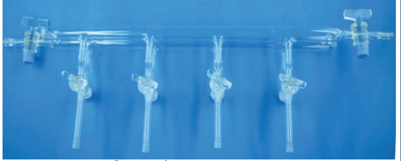
ÖZEL MANİFOLD CAM MUSLUKLU
